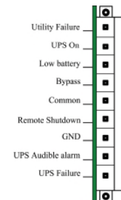
9-pin port
